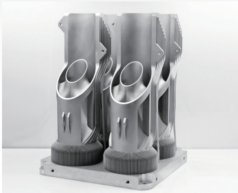
样品名称：智能水下机器人散热器 打印设备：FS301M 打印材料：FS AlSi10Mg
